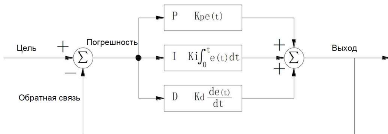
Рис. 5-20 Принципиальная схема ПИД-регулирования
