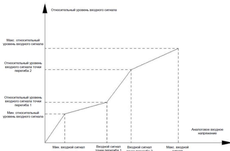
Рис. 5-17 Принципиальная схема настройки кривой 2/3
