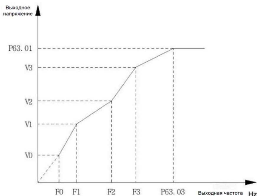
Рис. 5-6 Схематическая диаграмма многооточечной кривой вольт-частотного управления
